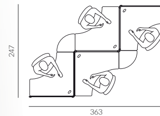
Ensemble composé de plateaux 90° 117 x 117 cm avec \frac{1}{4} de rond. Cloisons mixtes Mèlaminé / Polycarbonate et mixtes vagues Mèlaminé / Dual Satin. Plateaux Chêne de Fil Naturel (M) ou (S) CFN et Blanc (M) ou (S) BM.
