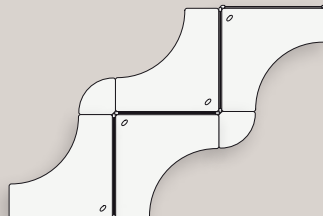
(423 x 287 cm) Réf. KSC 51
